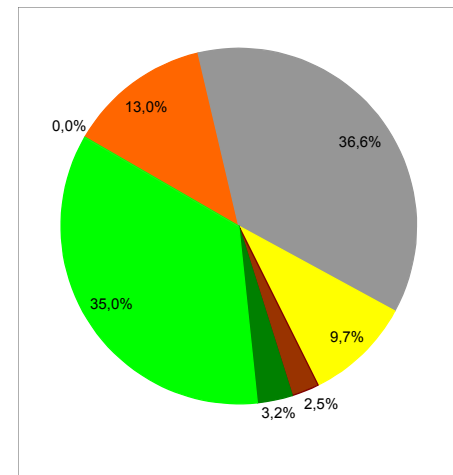
Stromerzeugung 2018 in Deutschland - Durchschnittswerte zum Vergleich
